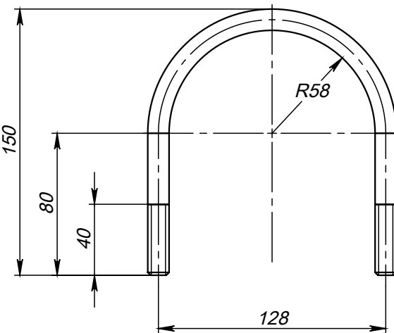
Поз.5 (Хомут)
